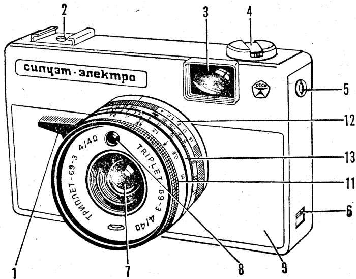
Рис. 1. Вид спереди
