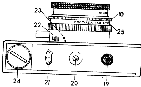
Рис. 3. Вид снизу
