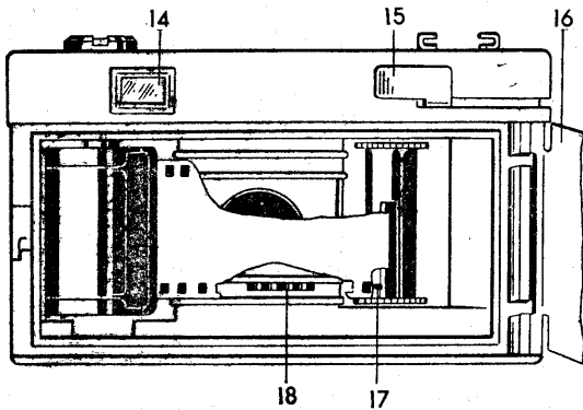
Рис. 2. Фотоаппарат с открытой задней крышкой
